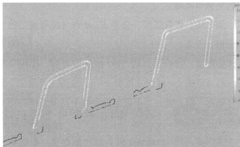
图 4 截面线偏差分析结果
