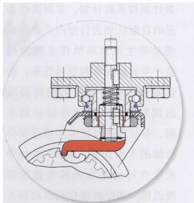
图 2 自动制动转向轮重要零部件的结构如图所示, 其中红色部分表示的就是 Progressus 公司研发生产的创新型自动制动机构
