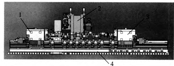
图1 HTM125600整机结构布局
