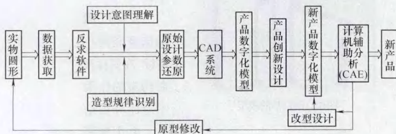
图1 逆向工程基本工作流程
