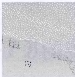
图4 删除非连接项
