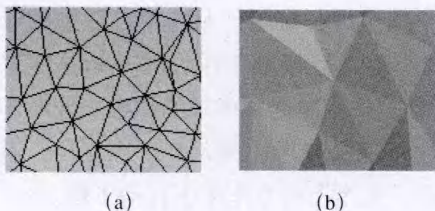
图7 三角形面片
