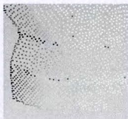
图5 删除体外孤点
