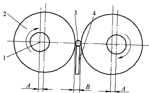
1.回转主轴 2.滚丝轮 3.工件 4.托板
