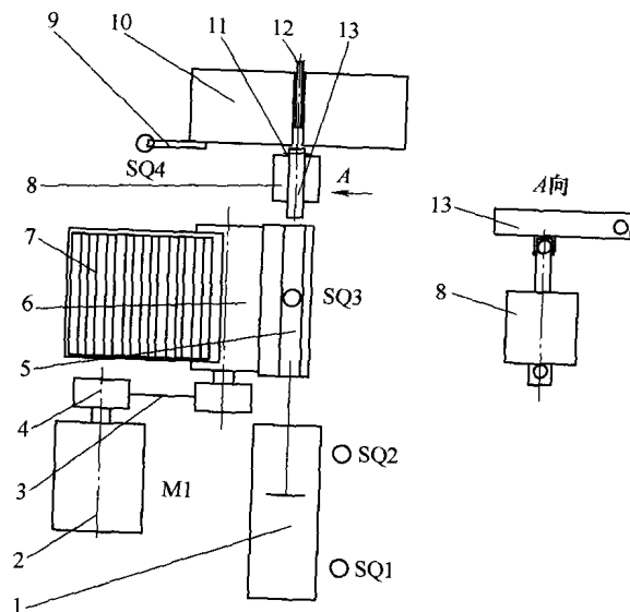
1.顶料气缸 2.送料电动机 3.传送带 4.带轮 5.下料槽 6.下料轮 7.料仓 8.下料气缸 9.长板 10.滚丝轮 11.铰链 12.定位板 13.托料槽
