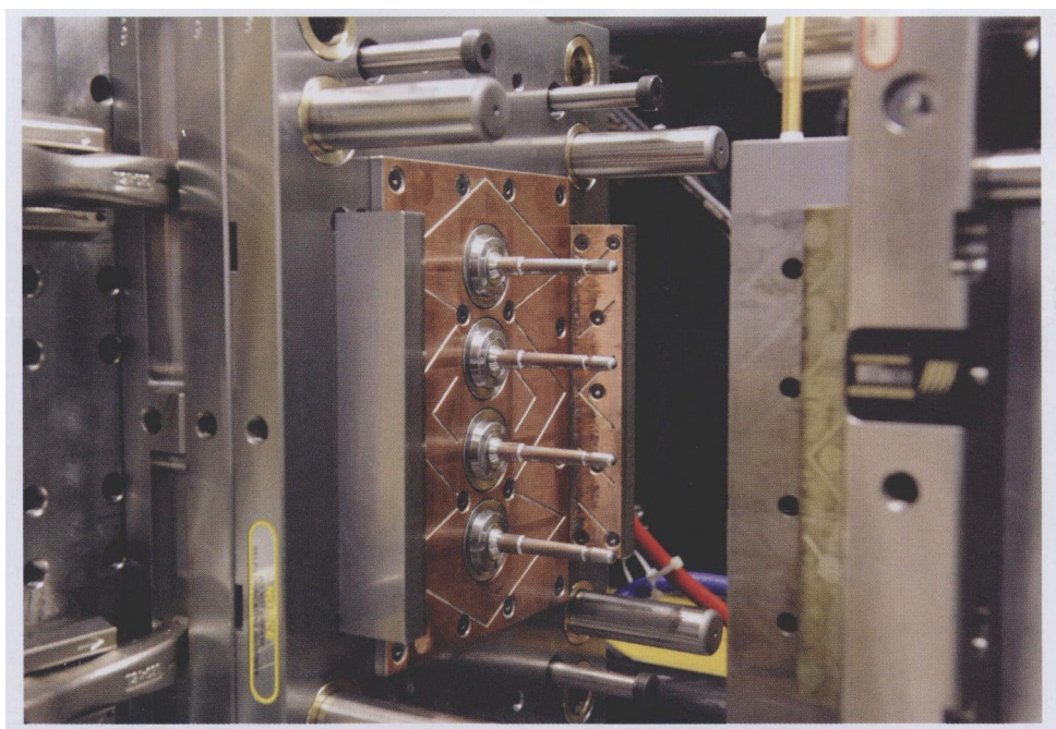
图中所示为由 Micron Products 公司制造的一套 4 型腔、高生产率的医疗模具
