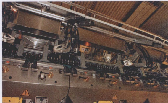
图 2 SIRIUS 3SE5 塑料型行程开关对食品行业使用的强力清洁剂尤具耐受能力。由于防护等级高达 IP66/67，工厂能够采用蒸汽喷吹的方式清洁设备
