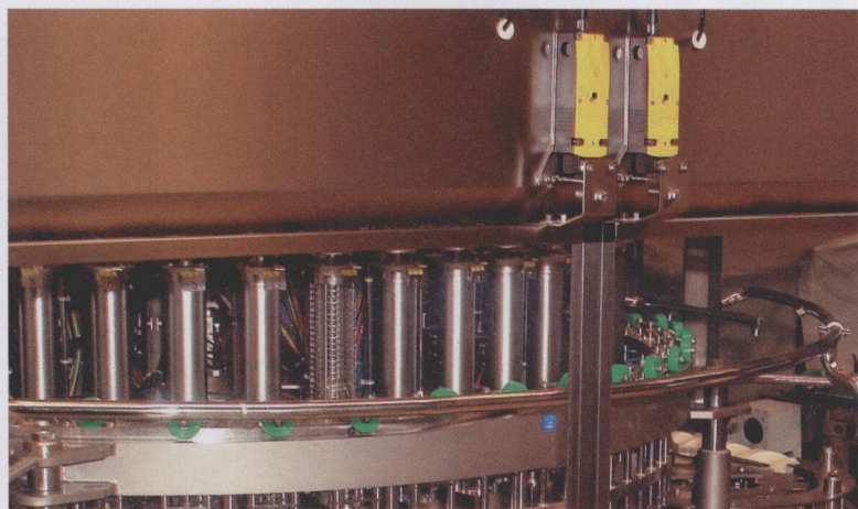
图 1 德国 Krones 工厂的安全解决方案根据 2006/42/EC 新机器指令进行了改造。西门子 ASIsafe 总线系统和 SIRIUS 3SF1 故障安全行程开关是预防风险的重要保护组件
