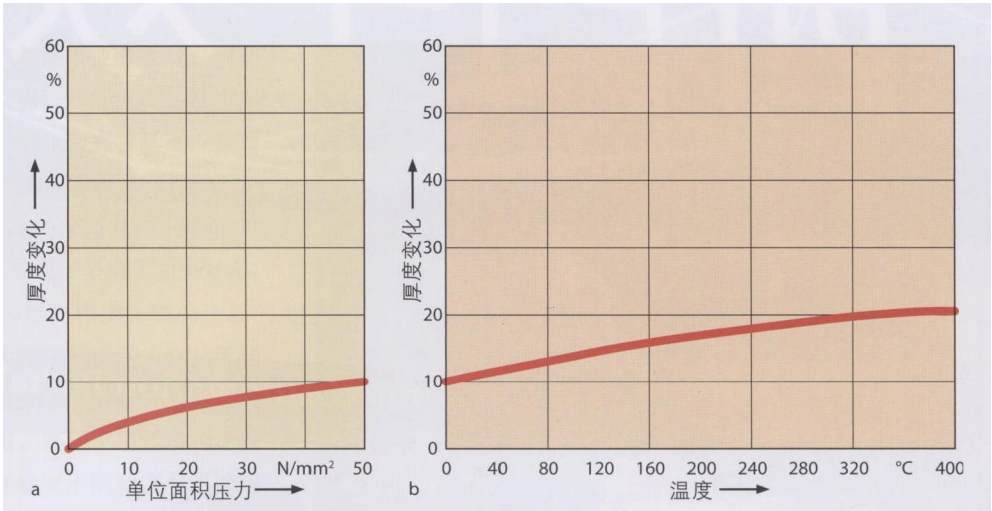
图2 在相同面积上使用更多的玻璃纤维会使密封垫更硬，蠕变性能下降，正如2mm厚玻璃纤维密封（HMF 15）收缩性能测试所表明的那样（A室温情况下；B单位面积应力50 N/mm²时）
