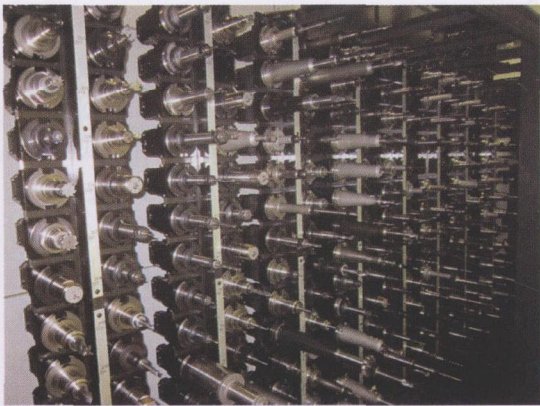
图 3: 基于每台机床的刀具库都拥有超过 200 个不同的刀具站，所以切削刀具库存的控制就具有关键性的意义。
