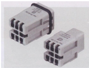
图 2 Harting 公司研制的 Han 7D 插塞连接器采用集成化快速锁合夹紧弹簧连接技术，因此在设备维护保养过程中可简单快捷地进行更换
