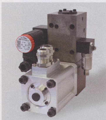
图 4 DECV 直驱式仿形电磁阀的工作原理与常规伺服阀截然不同，且没有敏感的先导控制油路，而是由伺服电动机直接驱动
