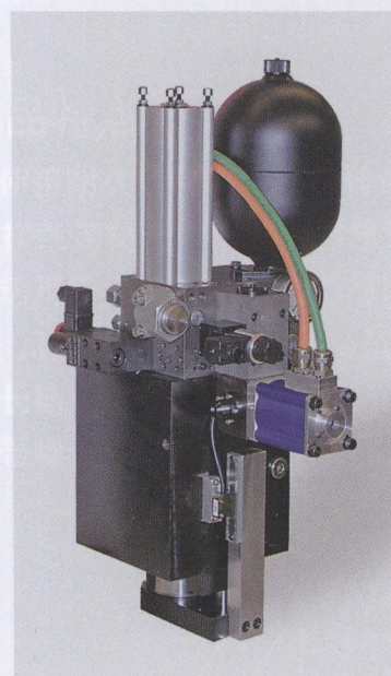
图3 适于在中等厚度板材成形加工领域使用的新型 HDM 液压驱动装置还满足了人们更高的需求，即步冲速度适度降低
