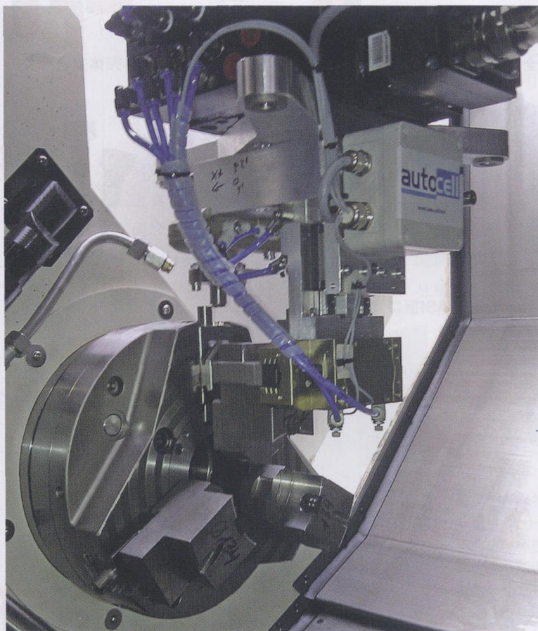
图 1 该车削加工单元首次实现了借助于机器人和 9 个专用夹钳自动更换刀具和刀具夹板
