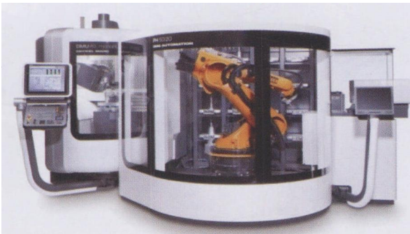
图 2 6 轴机器人型机床上下料生产线
