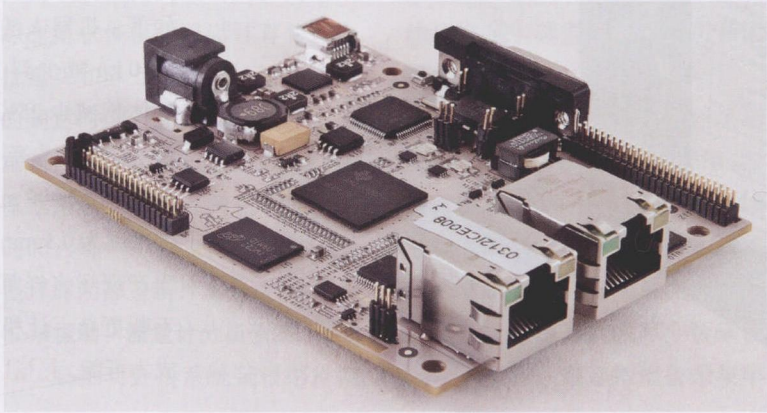
图 1 ICE 模块是一个带有多个工业界面的信号交换计算机工作的补充件，除了 CAN 和 Profibus 外，可支持各个通过软件定义的网络实时以太网通信协议 (Ethercat、Powerlink、Profinet)
