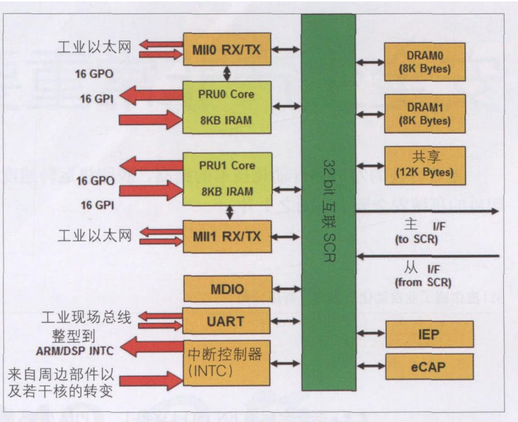
图 2 AM335x 里的 PRU-ICSS 子系统结构示意图
