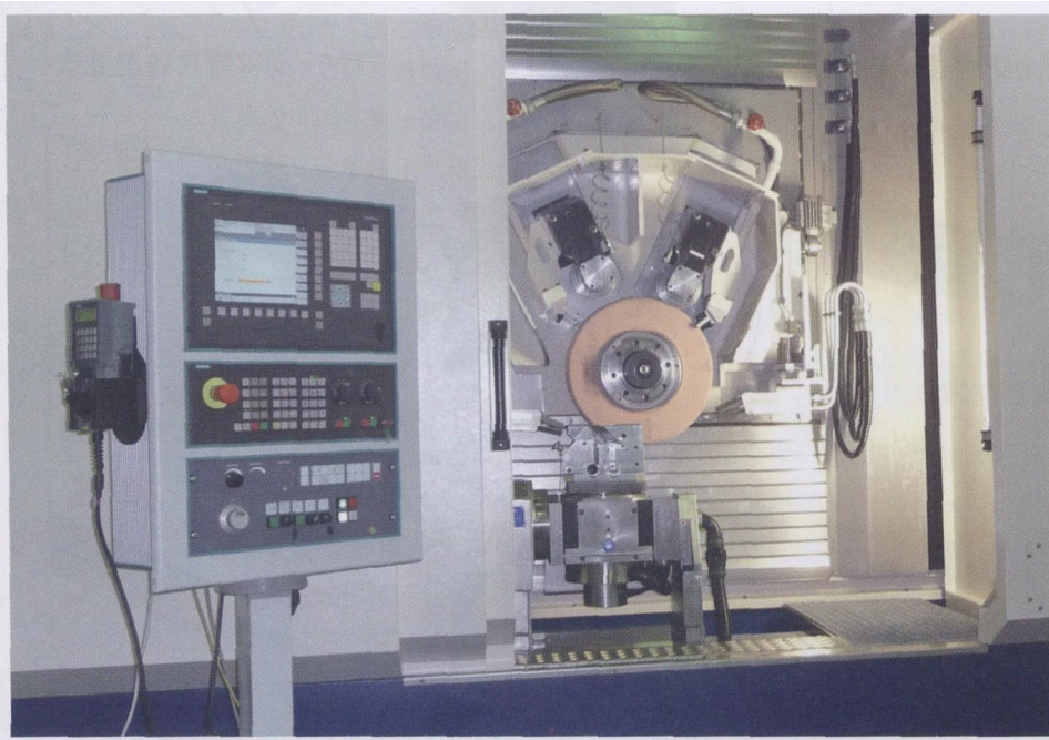
图1 适用于小批量涡轮叶片研磨加工作业的 Micro-Cut 4 520 S 型单螺杆磨床。画面右侧是砂轮件，砂轮后面是自动化砂轮更换装置
