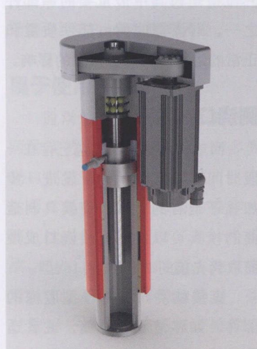
图3 由伺服电动机驱动的机电一体化的行星滚柱丝杠有着很大的驱动力同时又有非常紧凑的结构
