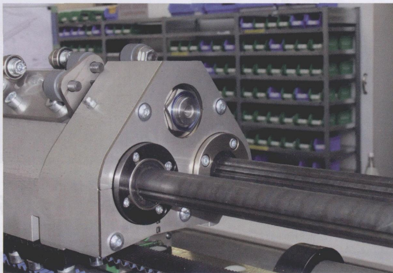
图 1 滚珠丝杠传动机构能够非常快速的传递很高的扭矩
