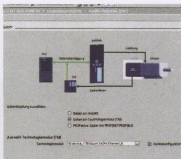
图4 简单且图示化实现机动控制组态
