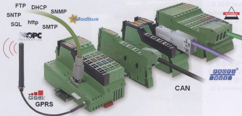
图 2 100 系列小型控制系统支持多种现场总线和 IT 标准
