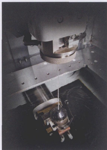
图 2 MV 系列经重新设计的自动穿线器能够在有或没有射流帮助的条件下实现切割线穿引操作
