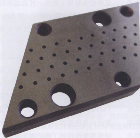
图 5 Mauer 将这个用于带孔压模的镶件作为一种将会受益于 MV 机床更可靠自动穿线器的部件实例。这个部件中心孔最初的测量值为 0.030 in, 然后经线割至最终 0.041 in
