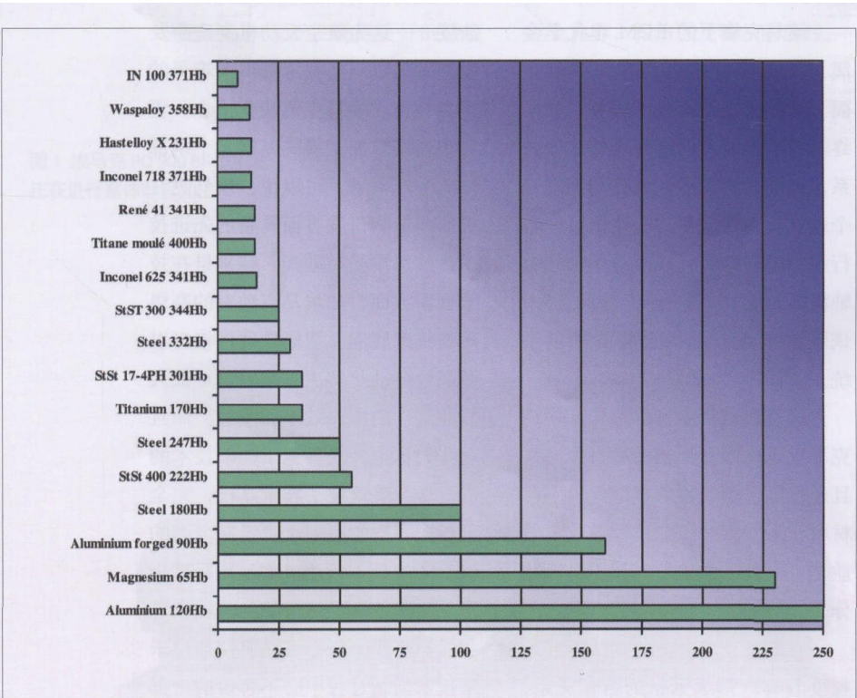
图 1 各类材料的难加工系数
