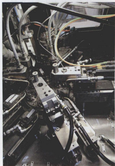
图 2 沟槽滑架与 横向刀架呈 V 形 分布在各工作主 轴旁，能可靠地 同时进行多种操 作
