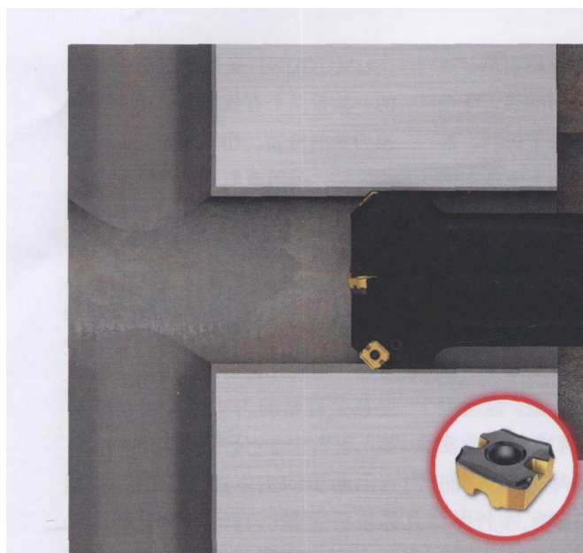
图2 伊斯卡采用专为加工高温合金而研制的 ISO 系列 SNMG 432-EM-R 硬质合金刀片
