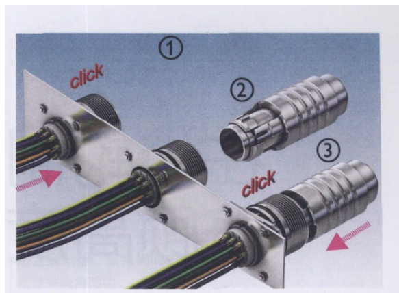
图3 Coninvers 公司研制的圆形连接器具有安装简便且工序安全可靠的特点，绝缘体可从后面啮合（如图中①所示），且可从正面解开（如图中②和③所示）
