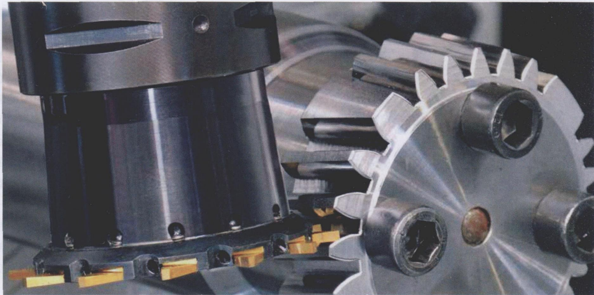
图 1 正在利用 InvoMilling 加工方法进行齿轮的加工
