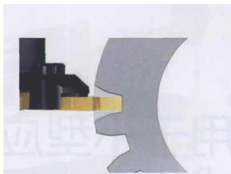
图 3 InvoMilling 方法将槽铣和车铣工序组合到一起。采用相同的刀具能够加工任意螺旋角的齿
