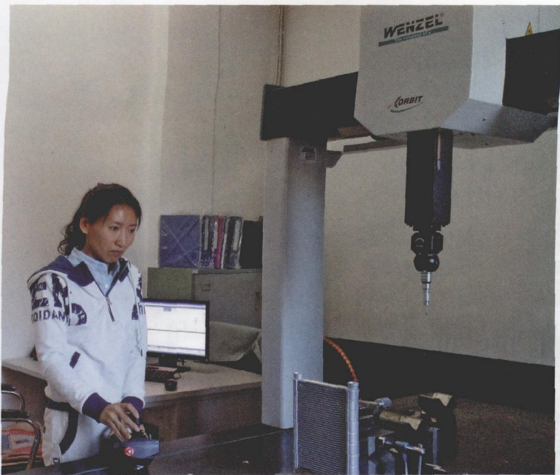
图2 孙晓佳正在操作温泽 XOrbit 系列三坐标测量机
