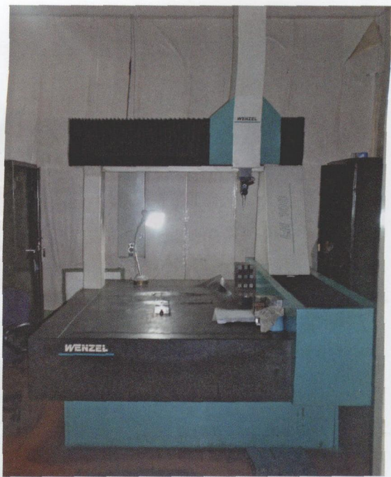
图3 服务于一汽集团已有 14 年的温泽 LH 系列三坐标测量机
