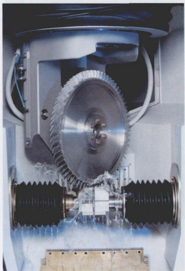
图 2 埃马克 PO 900 BF 加工区，采用精密电化学加工（PECM）技术进行整体叶盘的加工
