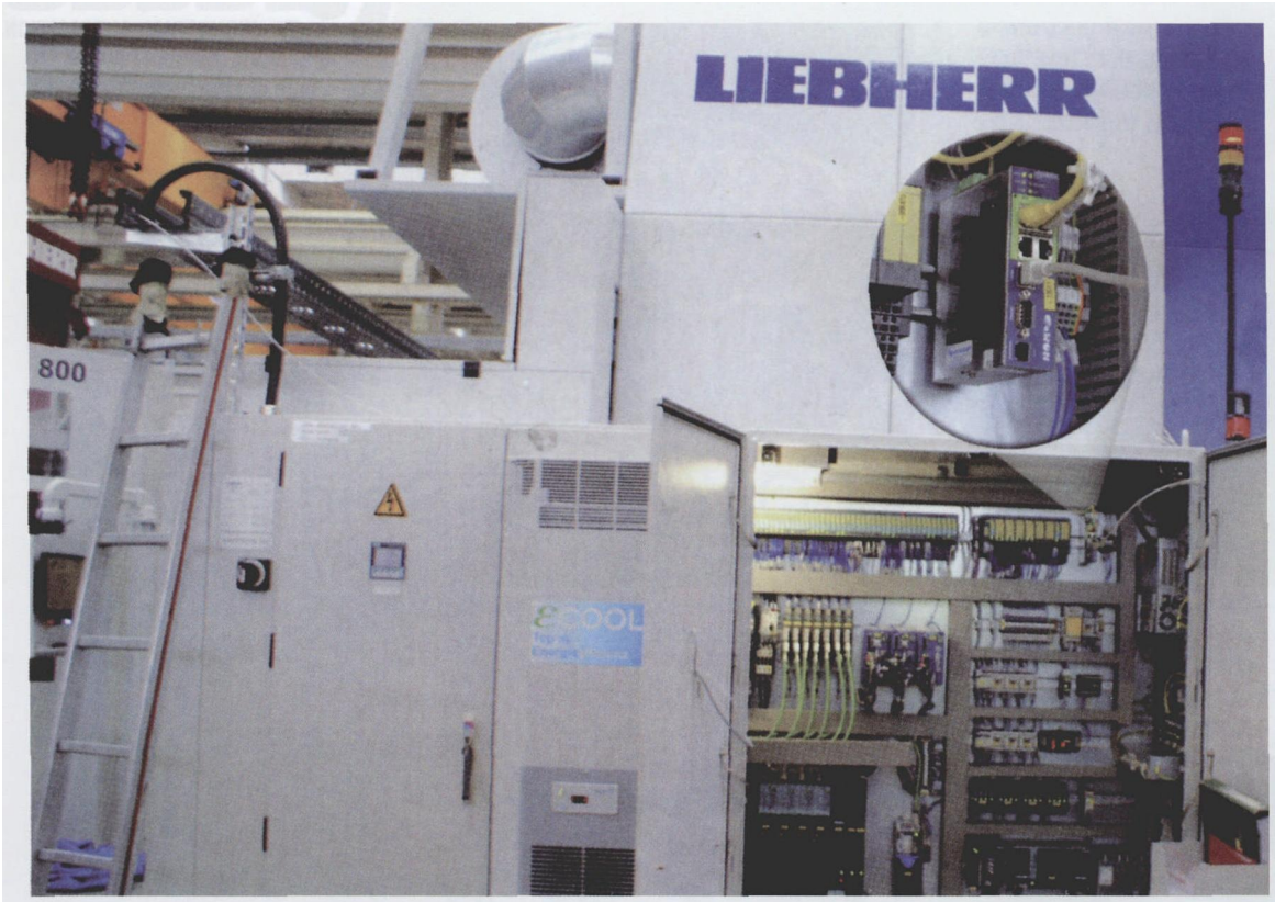
Wachendorff 的 eWON 系列远程维护路由器建立起了 Liebherr 公司与其所生产的在外界使用的设备的联系
