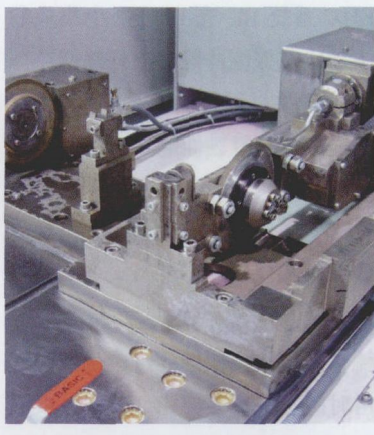
图 2 带有一体化冷却装置的金刚石辊的数控转动调节器
