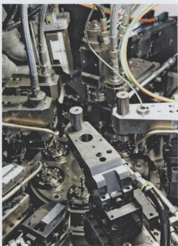
图2 沟槽滑架与横向刀架呈V形分布在各工作主轴旁，能可靠地同时进行多种操作
