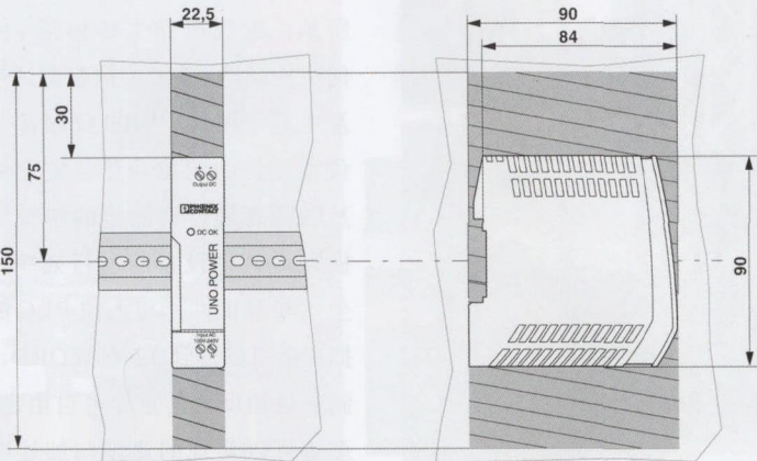
图 2 带标注尺寸的 Uno Power 供电装置
