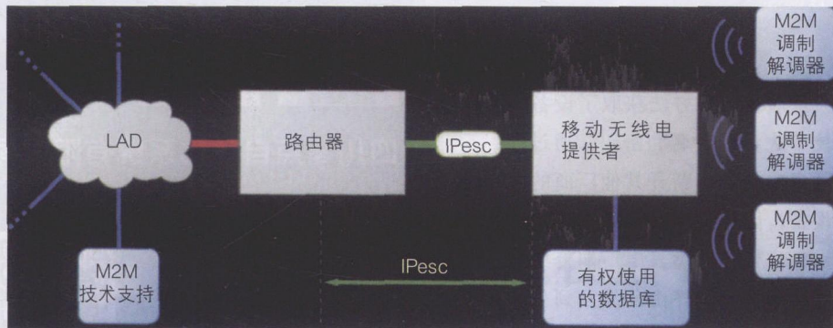
图 3 当由一个移动无线电提供者的基于 IPsec 的 VPN 基础设施可供使用时，问题不仅是缺少终端对终端的密码，还缺少虚拟的私人网络范围内的安全检验证实。对于要求功能安全的自动化应用而言，做到一个这样的技术解决方案是不成问题的
