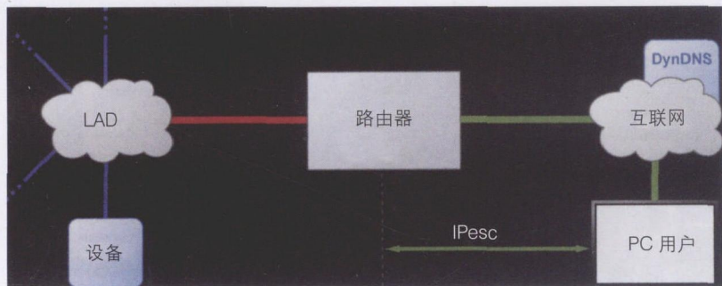
图2 有些技术解决方案也使用集成路由器 IPsec。在这种情况下,不存在终端对终端的编成密码,因为路由器中的 IPsec 结束,装置便可在不需要密码的情况下进行数据传递。因为在这样的远程信息存取技术解决方案中用预共享密钥进行工作,所以对于每个密钥的拥有者来说,均可进入 VPN
