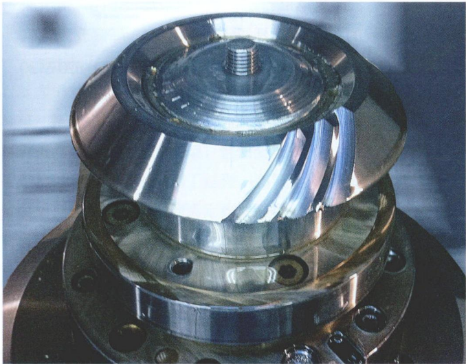
图 2 在深磨加工中锥齿轮毛坯：已经加工出 3 个缺口。Tandler 齿轮和传动装置生成厂可使用 Cubitron 11 型金属陶瓷研磨罐可在必须进行调整前大大加快更多缺口的加工制造
