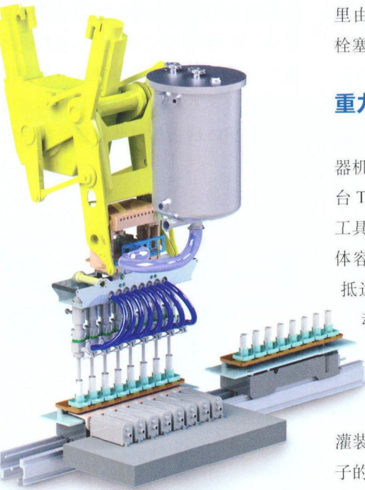
图3 TLM-F2 机器人支撑着带有灌装针的液体灌装工具。通过采用机器人技术既可防止灌装的液体超出规定平面，又可避免所灌装的液体低于规定平面
