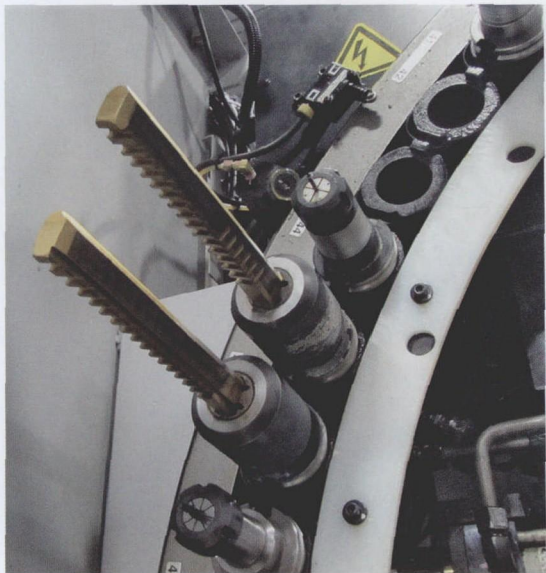
图2 卧式加工中心整合推削加工是可行的，因为推削刀具可以装到刀库中，并作为拉刀使用
