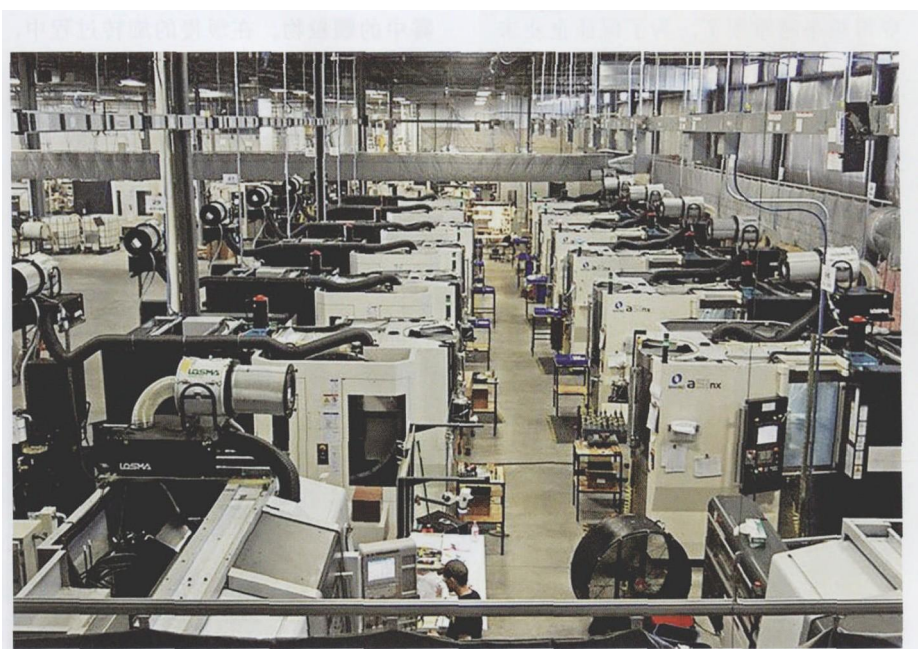
图 1 由 32 台 Makino a51nx 卧式加工中心组成的生产线，机床在相同的指导原则下运行，注重细节，力求确保加工精度的一致性
