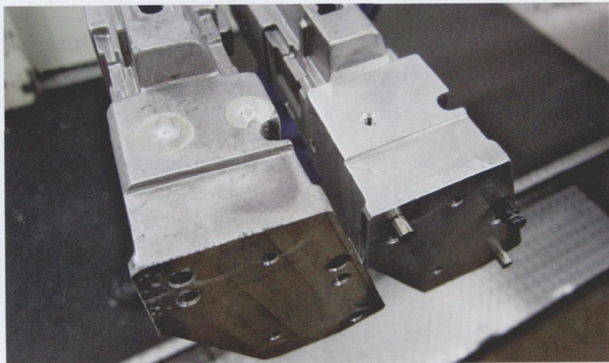
图 4 op.10 操作留下的粘合剂可通过 op.20 铣削操作移除
