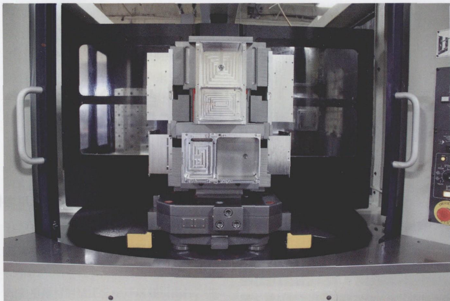
图2 Kiwa 的6托盘扩展加载站配备了立式夹具，能够在主轴正在执行其他任务加工时实现多个夹具装夹
