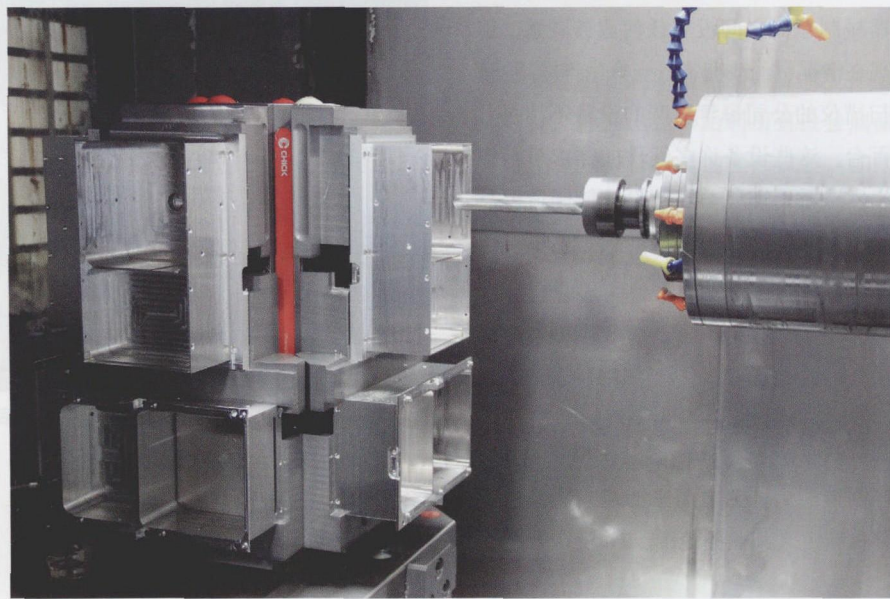
图3 Kiwa 卧式加工中心将此项任务的加工作业从4次减少到了两次，Baum 公司可就此最大程度地实现熄灯作业，而另外4个托盘仍然安装在机床上，开放给其他加工任务，并可以在前面任务正在执行时进行装夹
