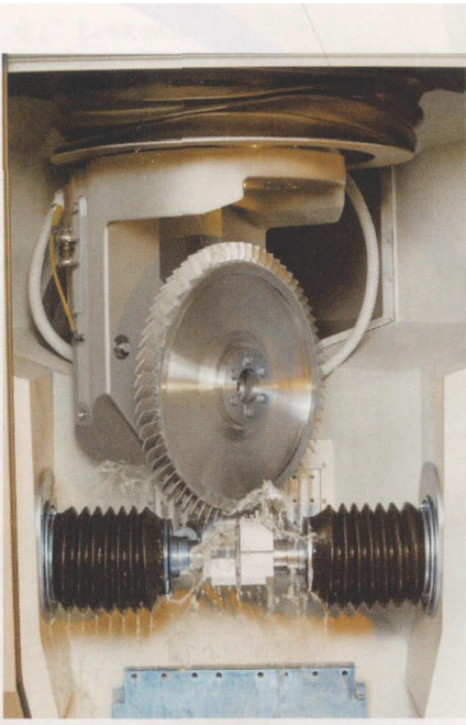
图1 埃马克 PO 900 BF 加工区，采用精密电化学加工（PECM）技术进行整体叶盘的加工
