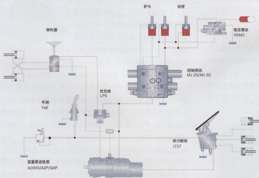
图 1：博世力士乐解决方案显著降低液压系统油耗
