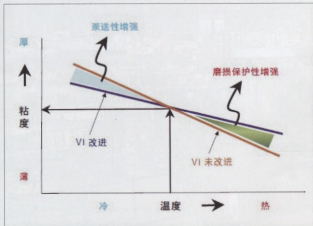
图2 高分子聚合物构成的添加剂能够较好地降低温度对粘度的影响
