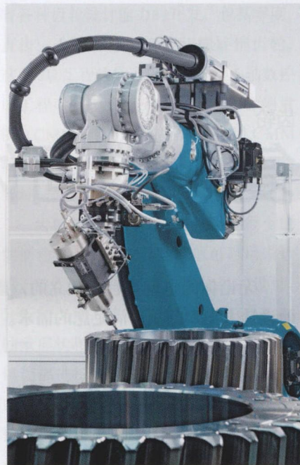
图4 作为一种机床的机器人，用于对钢质大型齿轮的边角轮廓进行加工：加工作业采用 VHM 铣刀，机器人能为轮齿加工出均匀的最大为 5 mm 倒角
