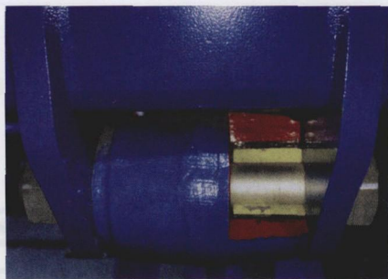
图1 这张图片展示了用在 Karat 9 的过冲元件轴套上的近乎黑色的 Iglidur G 型轴承
