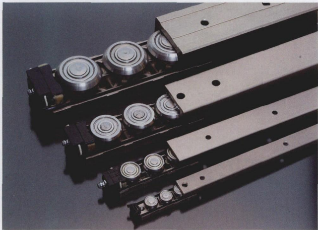
图 2 Rollon 的 Compact Rail 将滚珠轴承和滚道包含在滚子部件内
