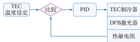
图3 激光器温度闭环控制示意图
