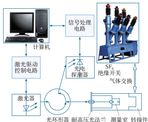
图8 TDLAS湿度测量装置结构示意图
