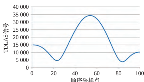
图10 加入匹配液后测量大气中绝对湿度的信号
