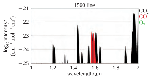
图2 1~2 \mu\text{m} 背景气中常见组分吸收谱线图
