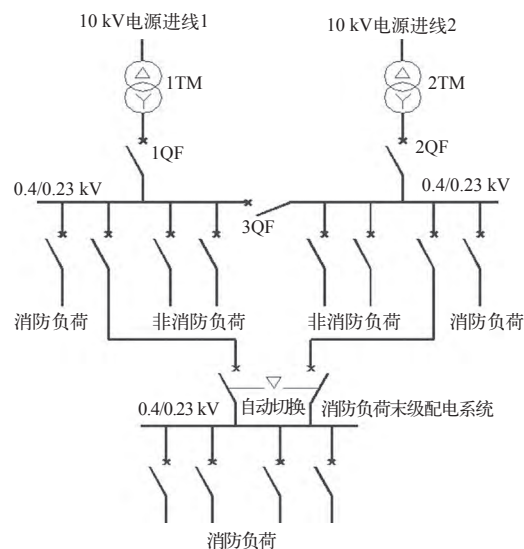
图1 常用供配电系统接线示意图
