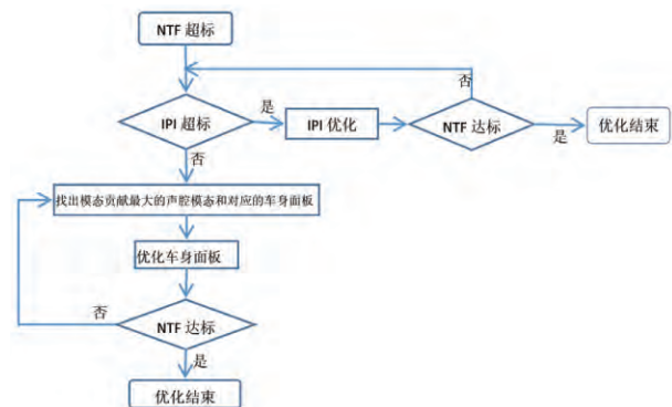
图 2 车身 NTF 优化流程
