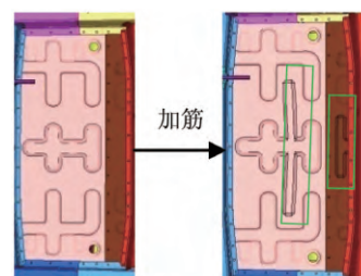
图 7 加强筋设计
