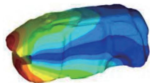
图 5 一阶上下模式 124.4Hz (第 7 阶)
