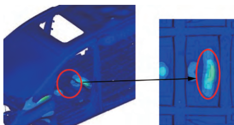
图 6 车身在前副后安装点 124Hz 的 ODS
