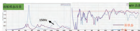
图 8 提高面板模式的改善效果
