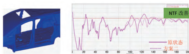
图 9 降低车身面板模式的改善效果
