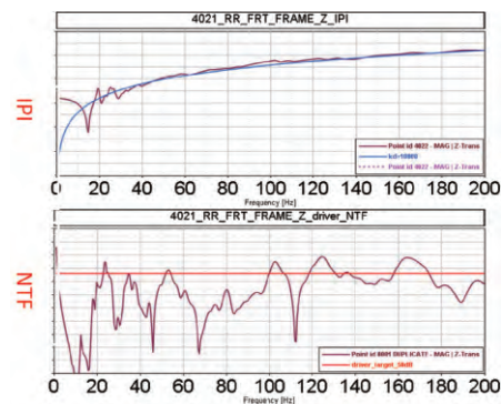
图 3 前副车架后安装点 IPI、NTF 分析结果
