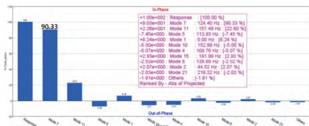
图 4 124Hz NTF 模式贡献量分析
