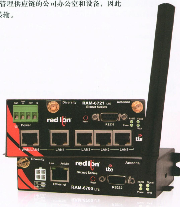
红狮控制 RAM 6000 蜂窝形路由器
