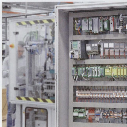
图2 系统集成商提供的安全子系统
