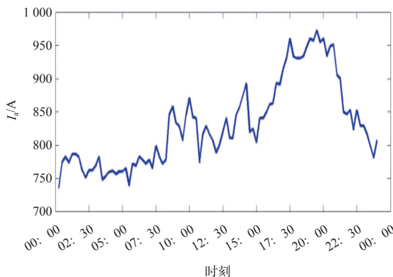
图5 某变电站主变压器电流曲线
