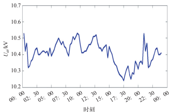
图4 某变电站母线电压曲线
