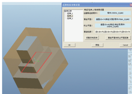
图8 工序特征构建界面
