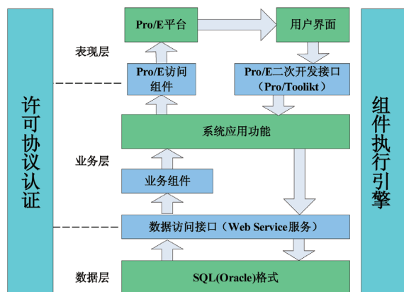
图 11 三维模型质量检测技术架构图
