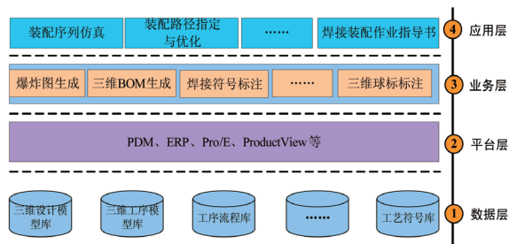
图 10 三维焊接装配技术架构图
