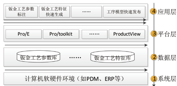
图9 三维钣金工艺设计技术架构图
